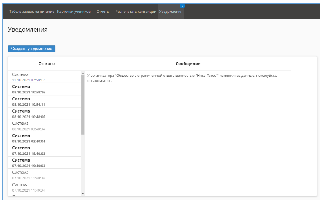
Рисунок 4.12 – Страница «Уведомления»
