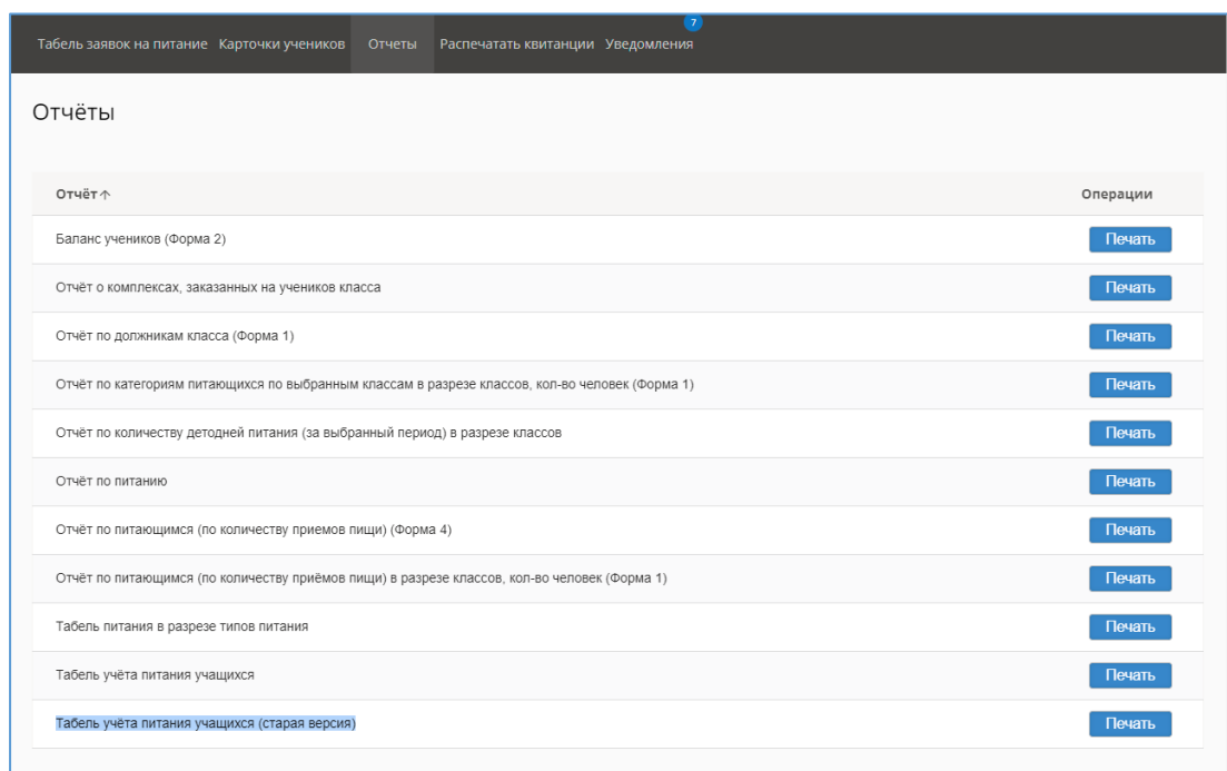
Рисунок 4.10 – Страница «Отчеты»
